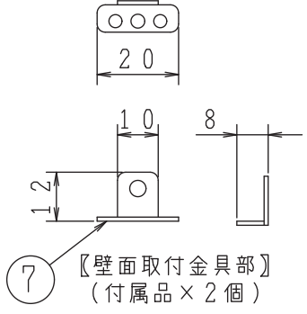
〔「壁面取付金具」取付イメージ〕
