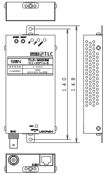
〔「壁面取付金具」取付イメージ〕
